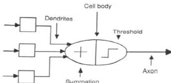
Slika 3-2 Umjetni neuron
