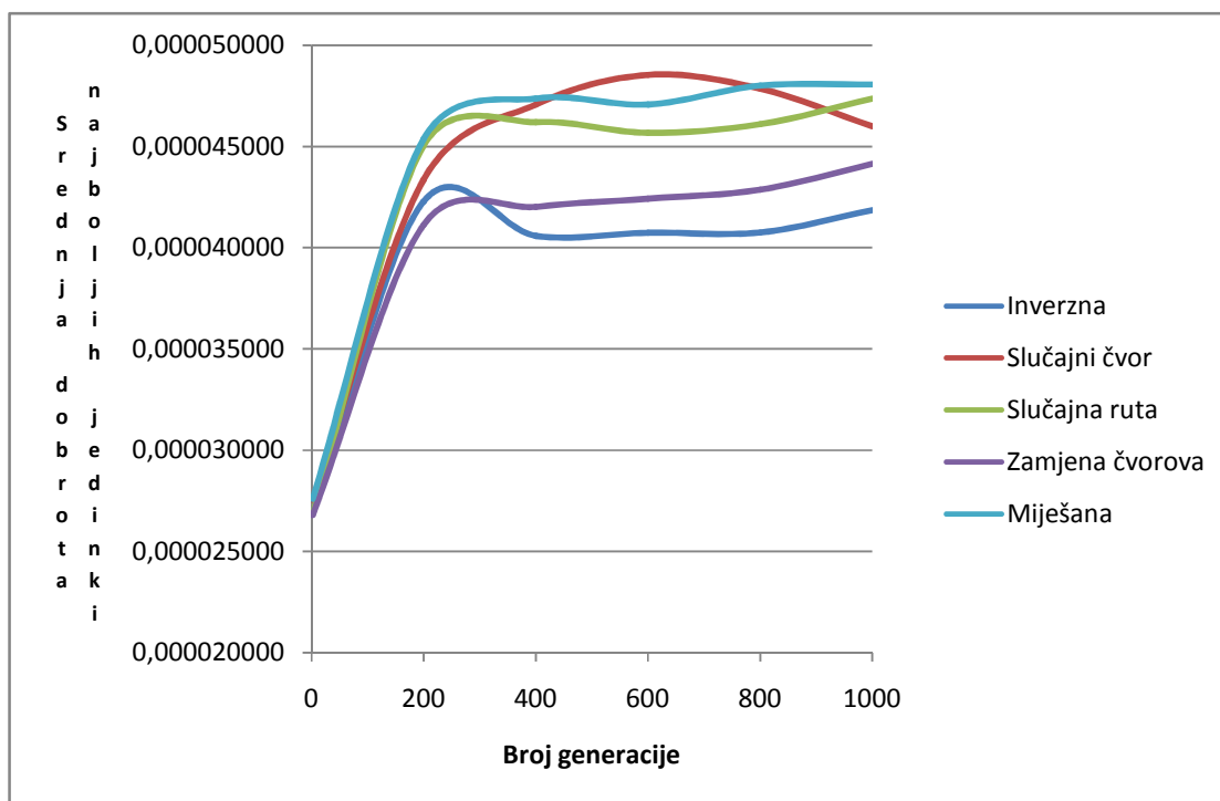
Slika 8.5 Graf srednjih vrijednosti najboljih jedinki u ovisnosti o odabiru različitih operatora mutacije
