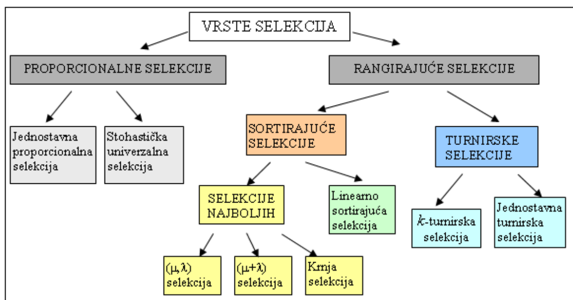
Slika 2.2 Podjela selekcija
