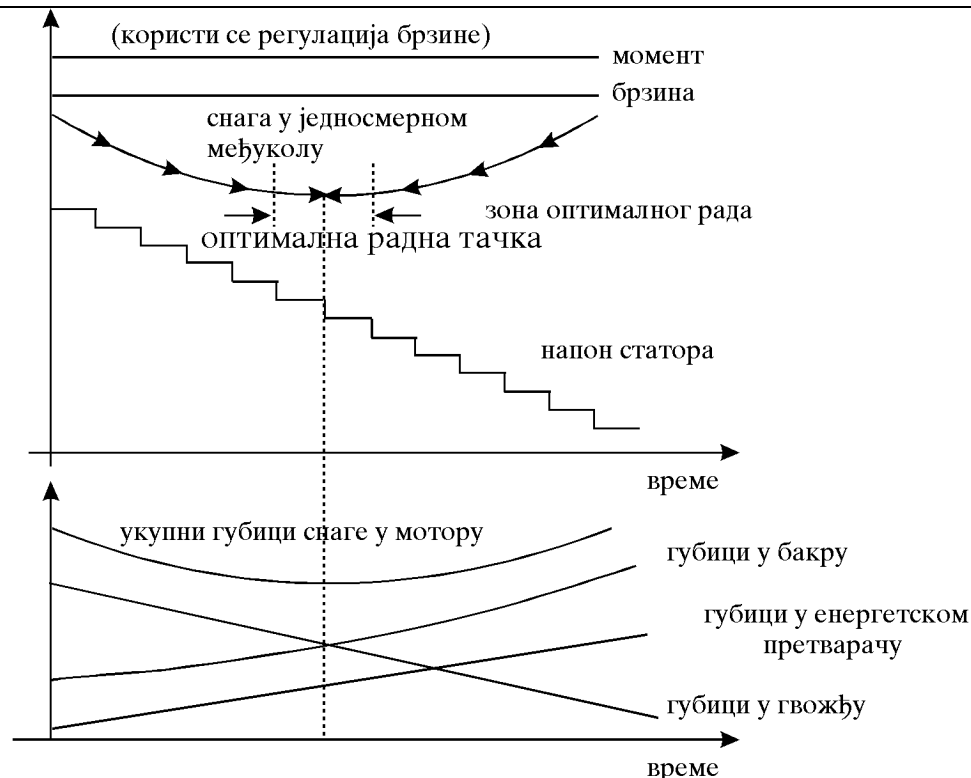
Slika 2.3.6.: Optimalno upravljanje variranjem statorskog napona.
