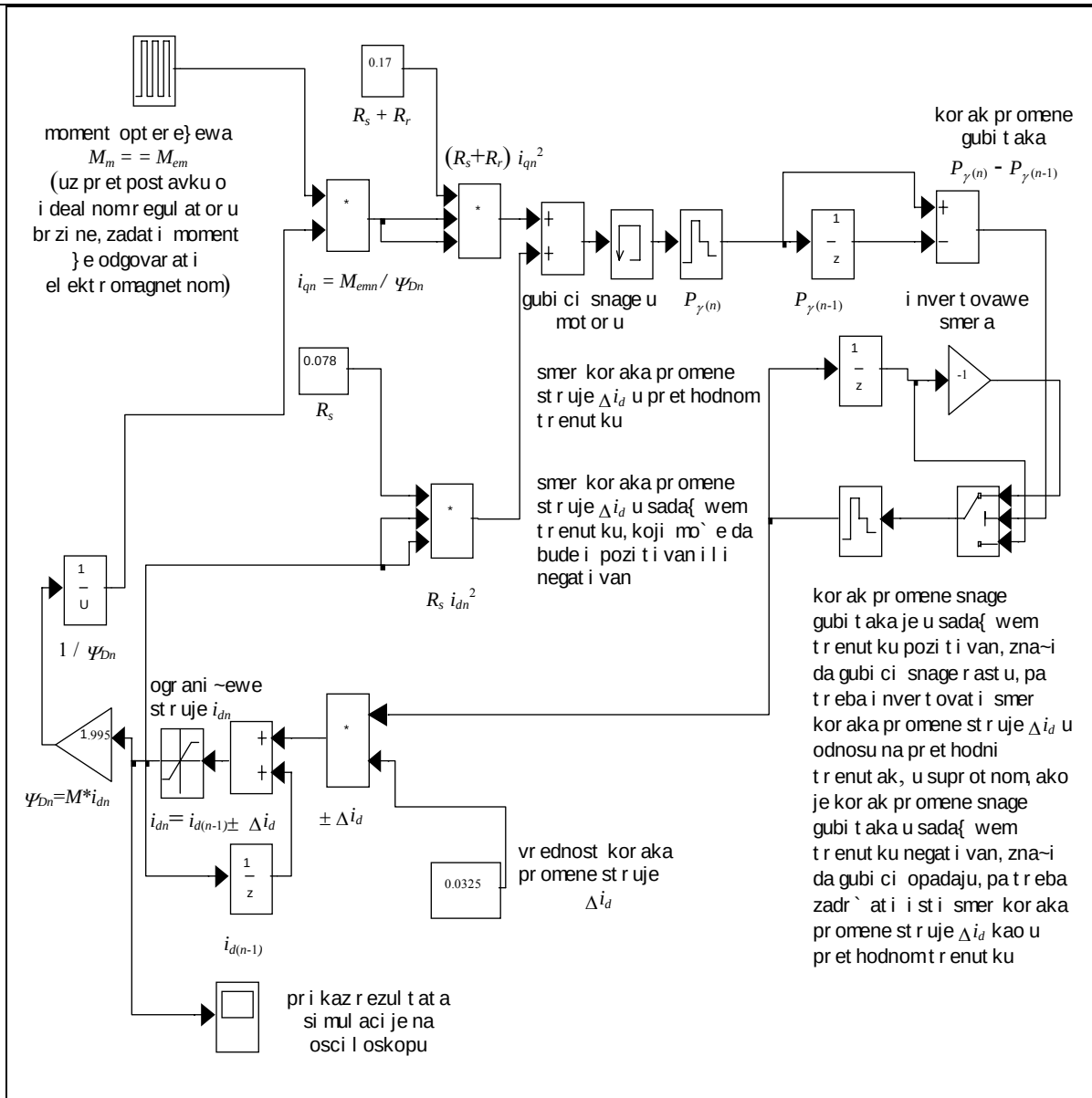
Slika 3.3.2.2.: Blok dijagram optimizacionog modela sa konstantnom veli~inom koraka promene struje i_d
