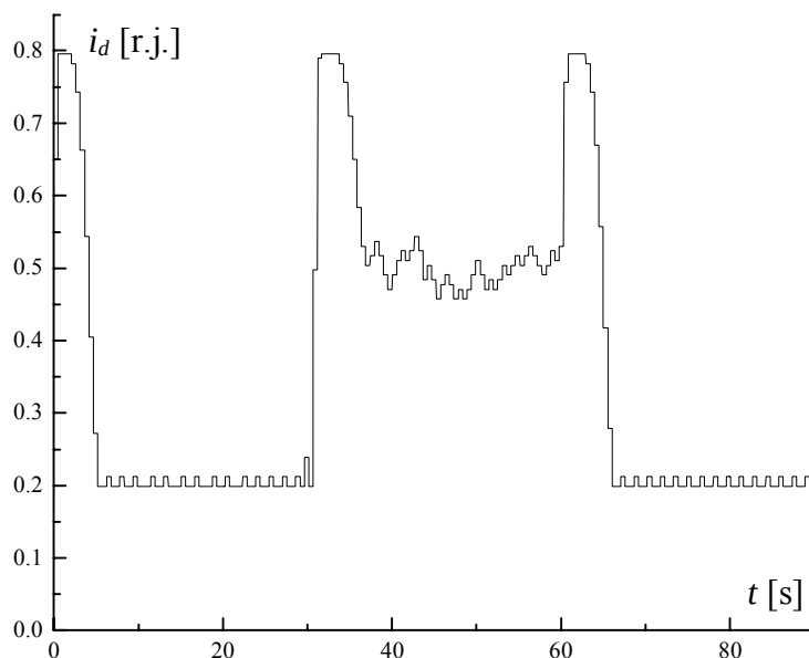
Slika 5.3.4. - 1, fazi optimizacioni algoritam, i_{dmin} = 2 \% , (grafik struje i_d , optimizira se P_{ul} , n = 400 \text{ ob/min} , M_1 = 0.03 M_n , M_2 = 0.7 M_n , M_3 = 0.03 M_n ).
