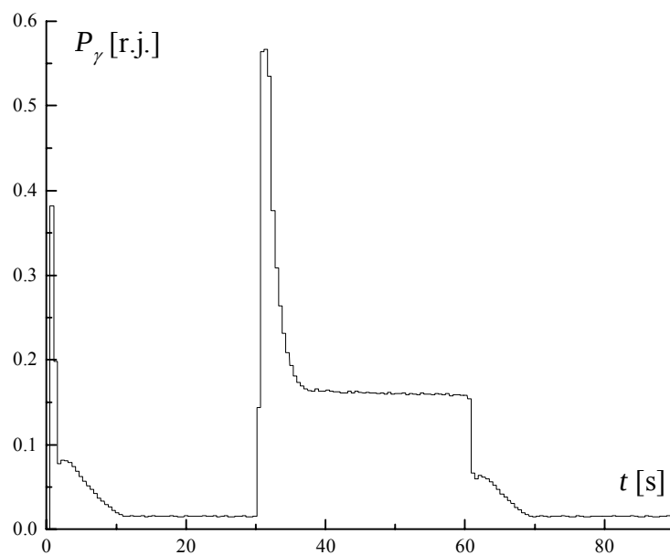
Slika 5.3.3. - 1v, višekoračni algoritam, i_{dmin} = 1 \% , i_{dmax} = 5 i_{dmin} , (grafik snage gubitaka P_\gamma , optimizira se P_\gamma , n = 400 ob/min, M_1 = 0.03 M_n , M_2 = 0.7 M_n , M_3 = 0.03 M_n ).
