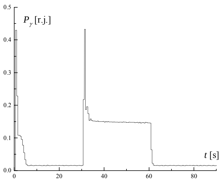
Slika 5.3.4. - 1v, fazi optimizaciji algoritam, i_{dmin} = 2\% , (grafik gubitaka snage P_\gamma , optimizira se P_\gamma , n = 400 ob/min, M_1 = 0.03 M_n , M_2 = 0.7 M_n , M_3 = 0.03 M_n ).
