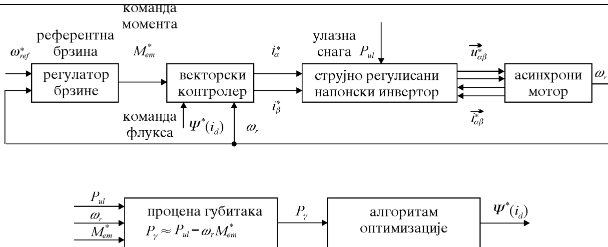
Slika 3.1.: Mehanizam prilagođavanja fluksa momentu opterećenja.
