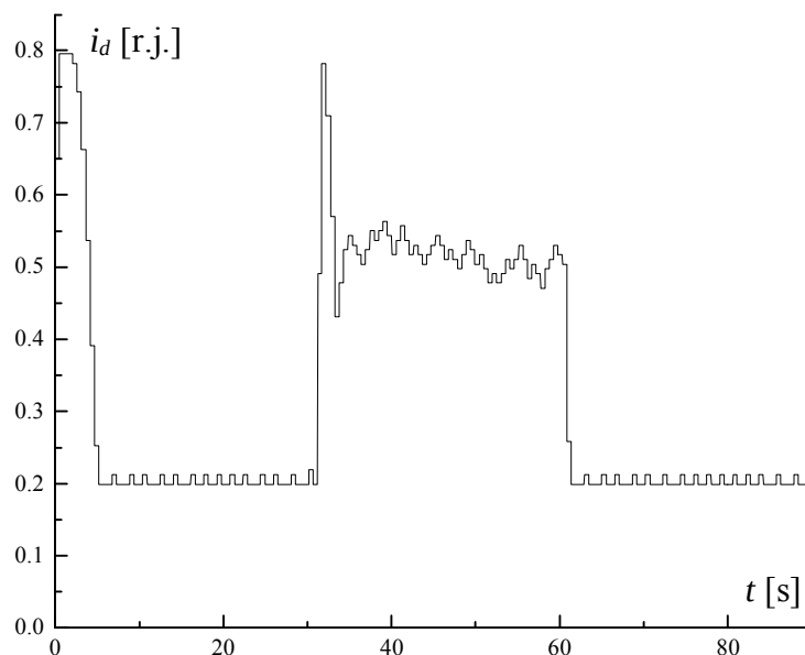
Slika 5.3.4. - 1a, fazi optimizacioni algoritam, i_{dmin} = 2 \% , (grafik struje i_d , optimizira se P_\gamma , n = 400 \text{ ob/min} , M_1 = 0.03 M_n , M_2 = 0.7 M_n , M_3 = 0.03 M_n ).
