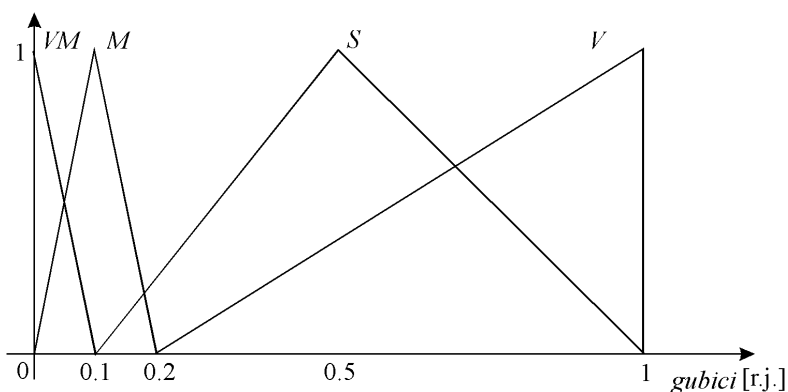
Slika 4.3.1.3.: Funkcije pripadnosti za opisnu promenljivu "gubici".
