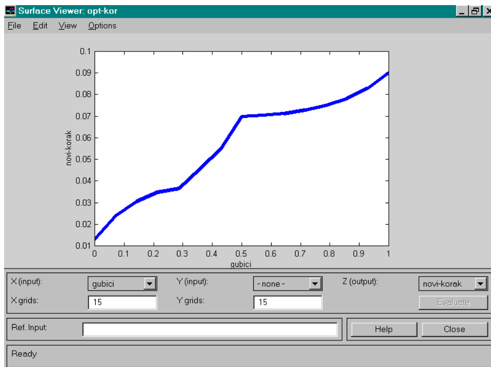
Slika 4.2.5.: Izgled ekrana za prikaz generisane upravjačke funkcije u Fuzzy Logic Toolbox - u, Matlab 5.0.
