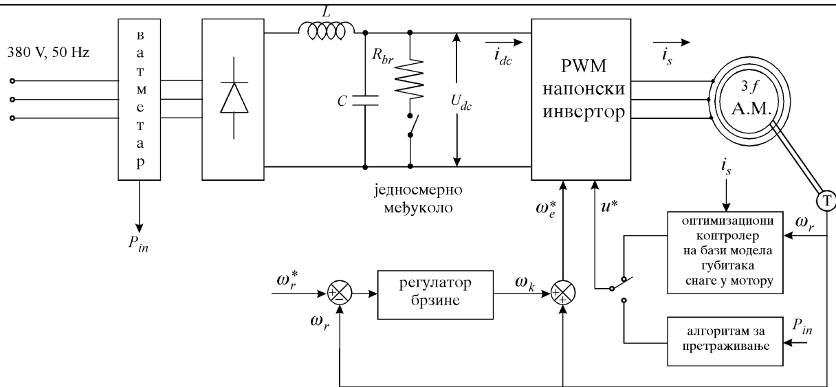
Слика 2.2.6.: Блок дијаграм управљачке структуре за оптимизацију степена корисног дејства скаларно управљаног погона.
