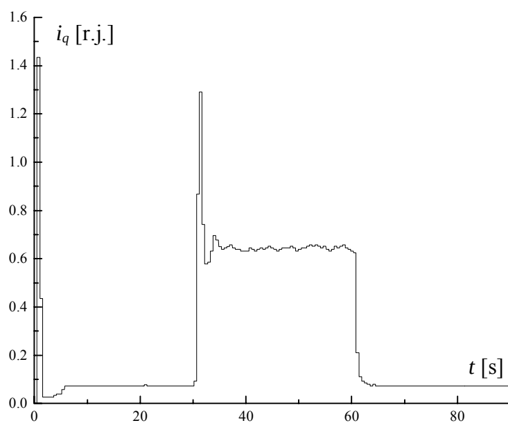
Slika 5.3.4. - 1b, fazi optimizaciji algoritam, i_{dmin} = 2\% , (grafik struje i_q , optimizira se P_\gamma , n = 400 ob/min, M_1 = 0.03 M_n , M_2 = 0.7 M_n , M_3 = 0.03 M_n ).
