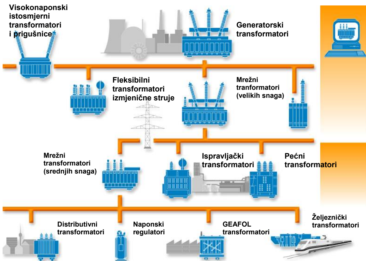
Slika 1-1: Podjela energetskih transformatora
