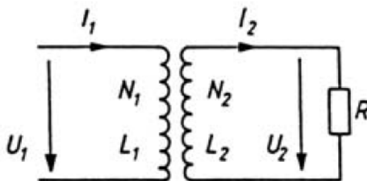
Slika 2-1: Idealni transformator
