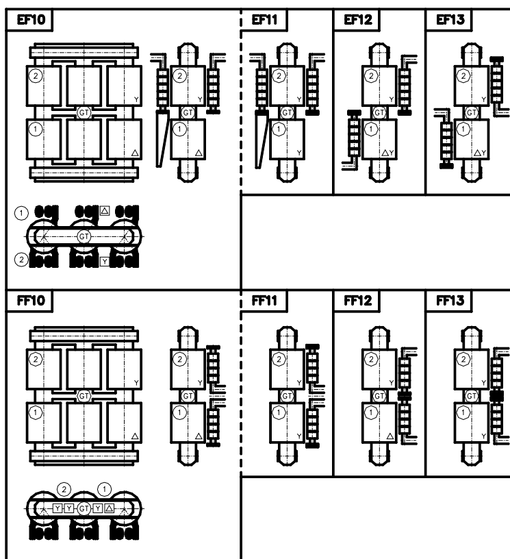
Tablica 2-9: Ispravljački transformatori (dvokatna izvedba)
