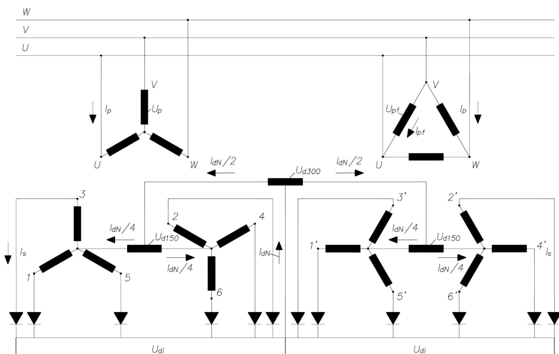
Slika 2-6: Spoj dvostruke zvijezde(sekundar) s usisnom prigušnicom
