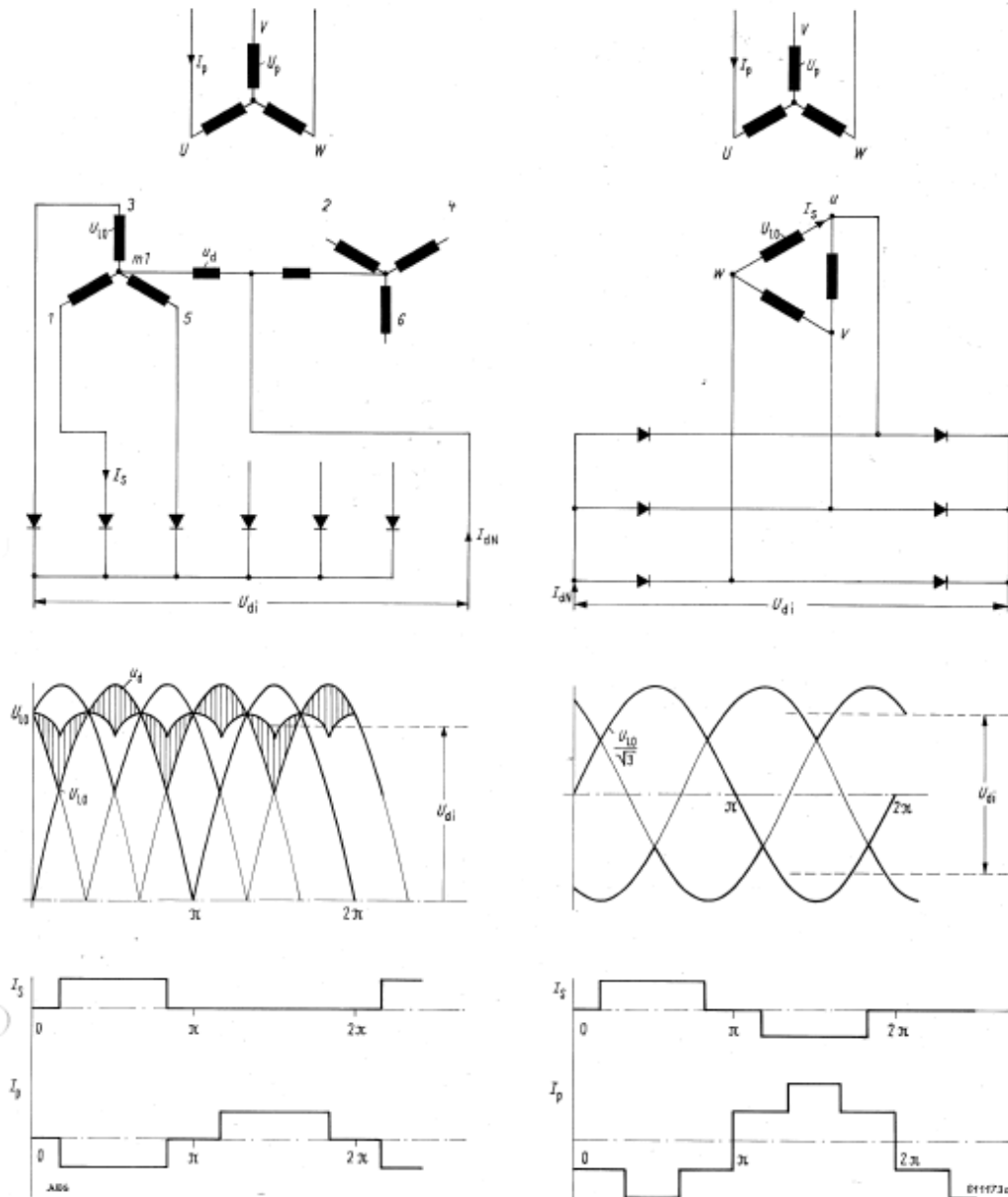
Slika 2-5: Ispravljački transformatori u poluvalnom DSS (lijevo) i punovalnom DB (desno) spoju
