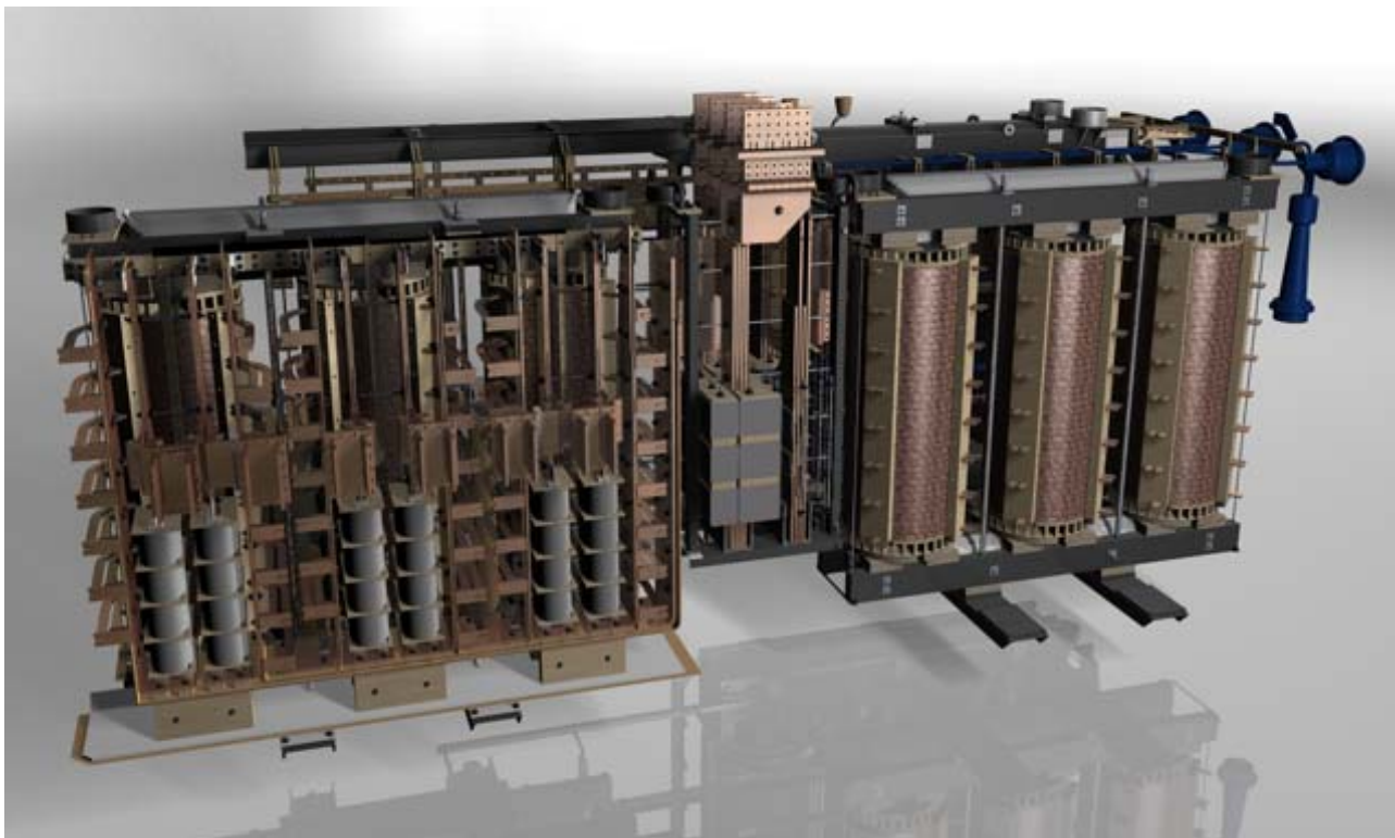
Slika 5-9: Aktivni dijelovi ispravljačkog transformatora
