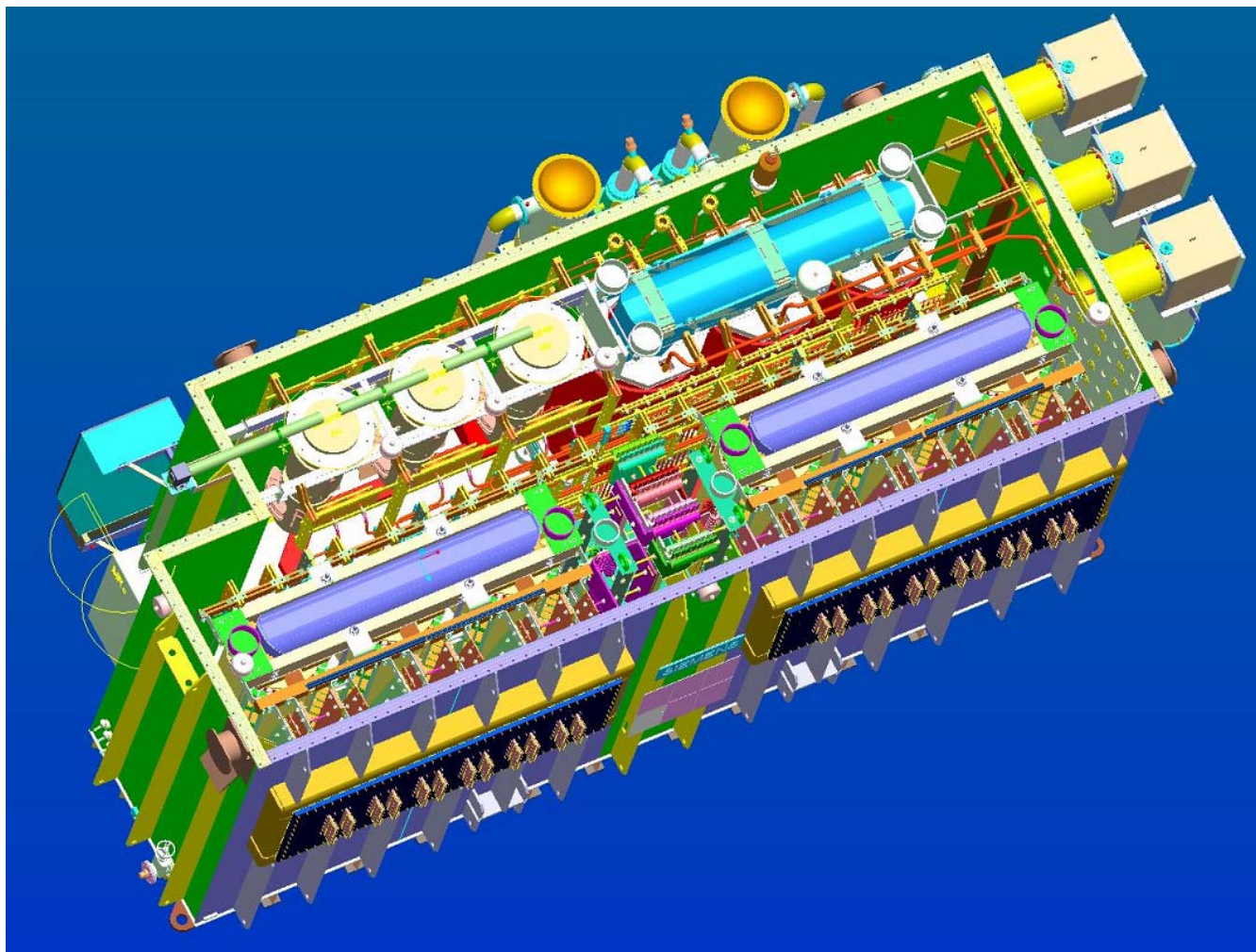
Slika 5-8: Projektno - konstrukcijsko rješenje (Model u ProE-u)
