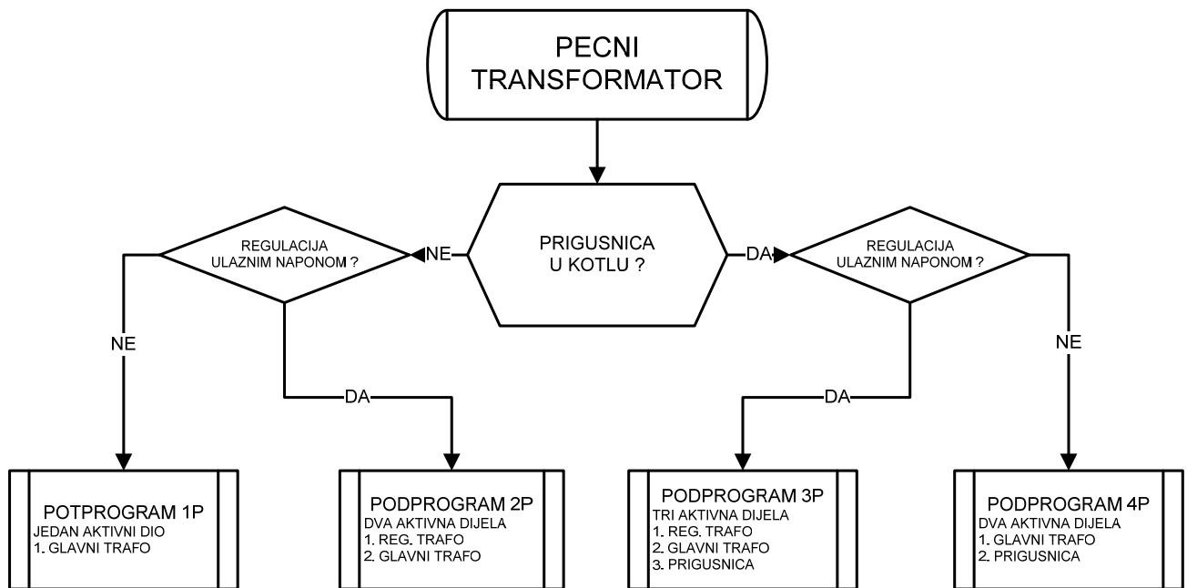
Slika 2-23: Dijagram toka pećnih transformatora
