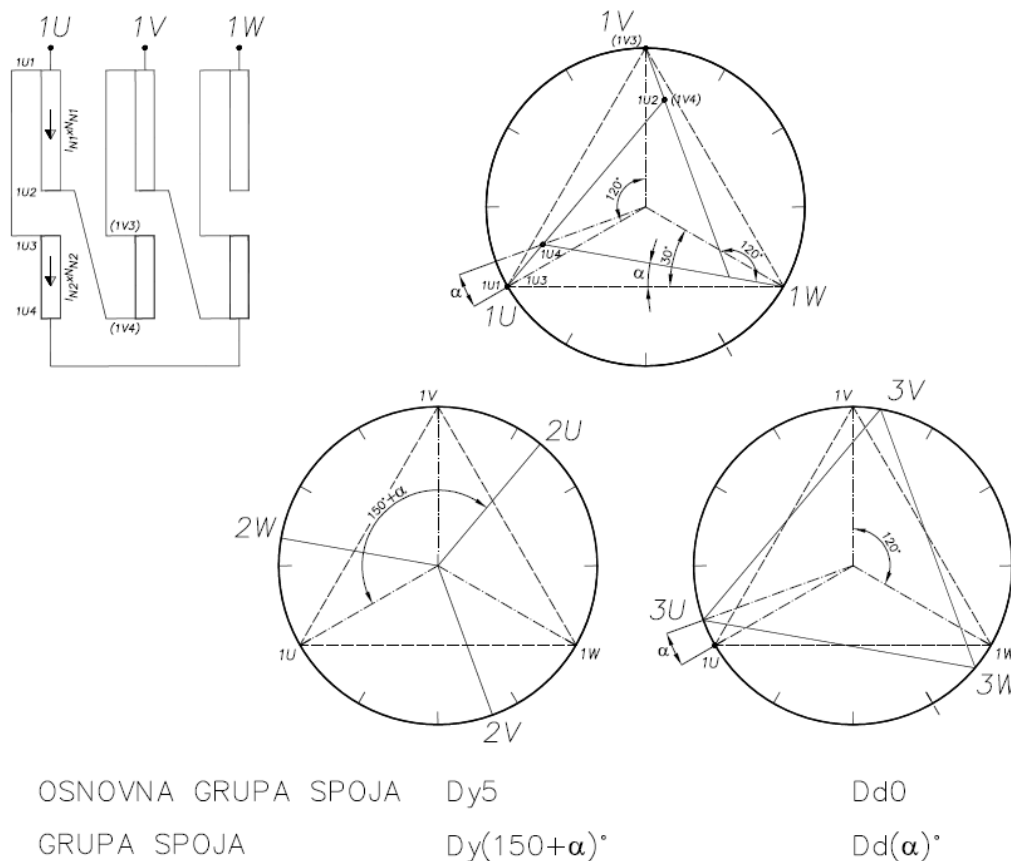
Slika 2-9: Produženi trokut kod „pozitivnog“ faznog pomaka za kut \alpha
