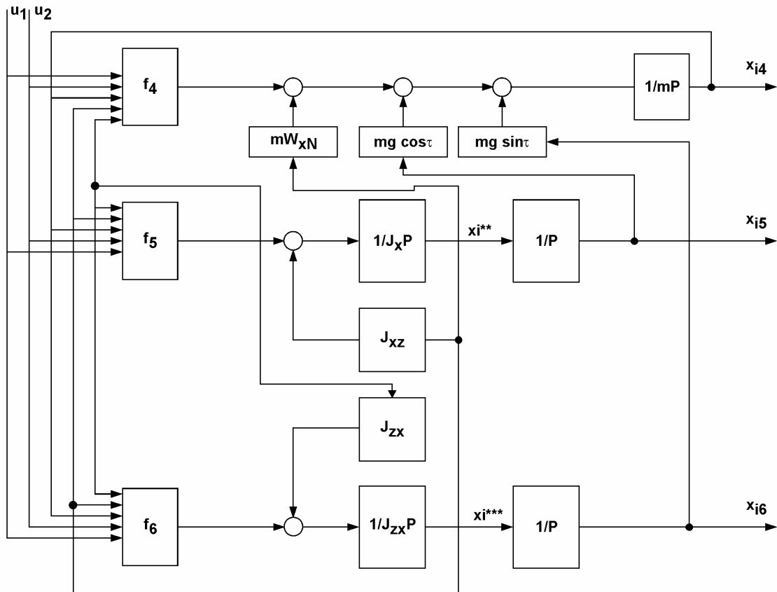
Sl. 8. Shema prečnega gibanja Fig. 8. Schematic for lateral motion
