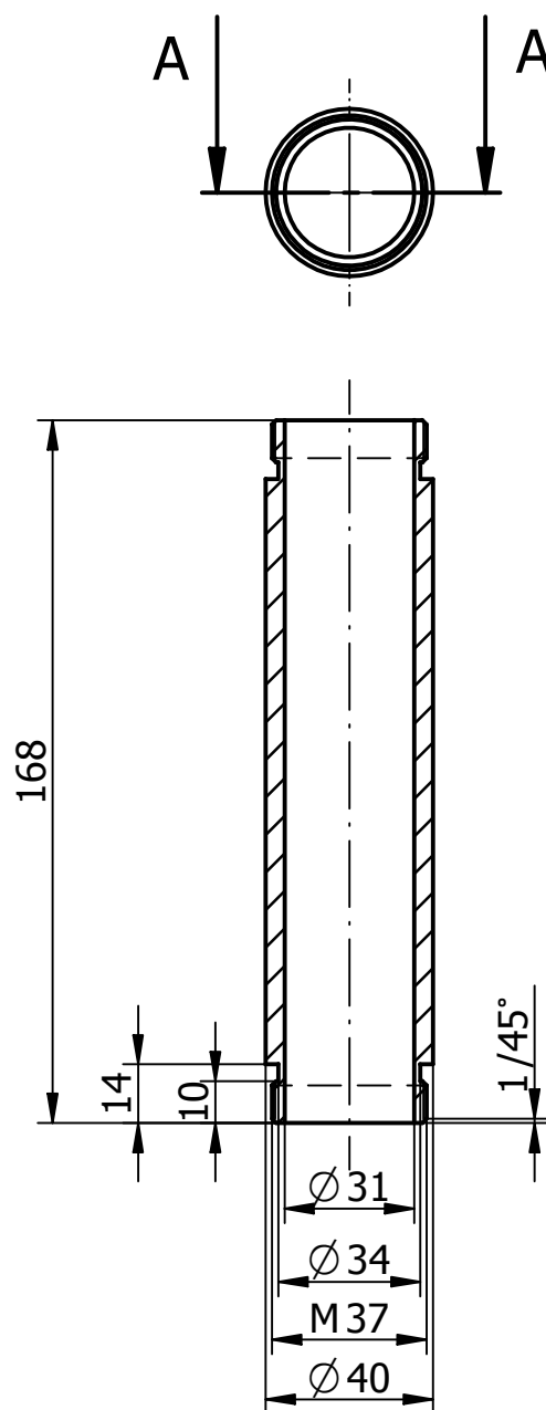
Presek A-A
