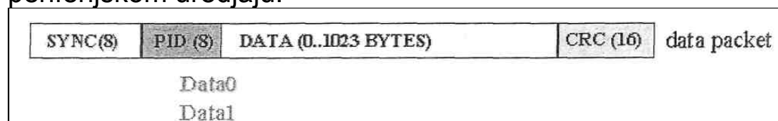
Sl.15. Format Data paketa
