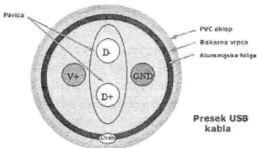
Sl. 1 Presek USB kablo
