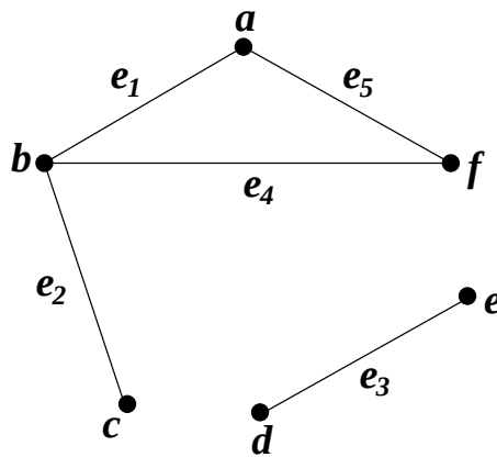
Slika 2.1. Neusmjereni graf.
