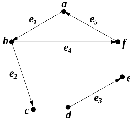
Slika 2.2. Usmjereni graf.
