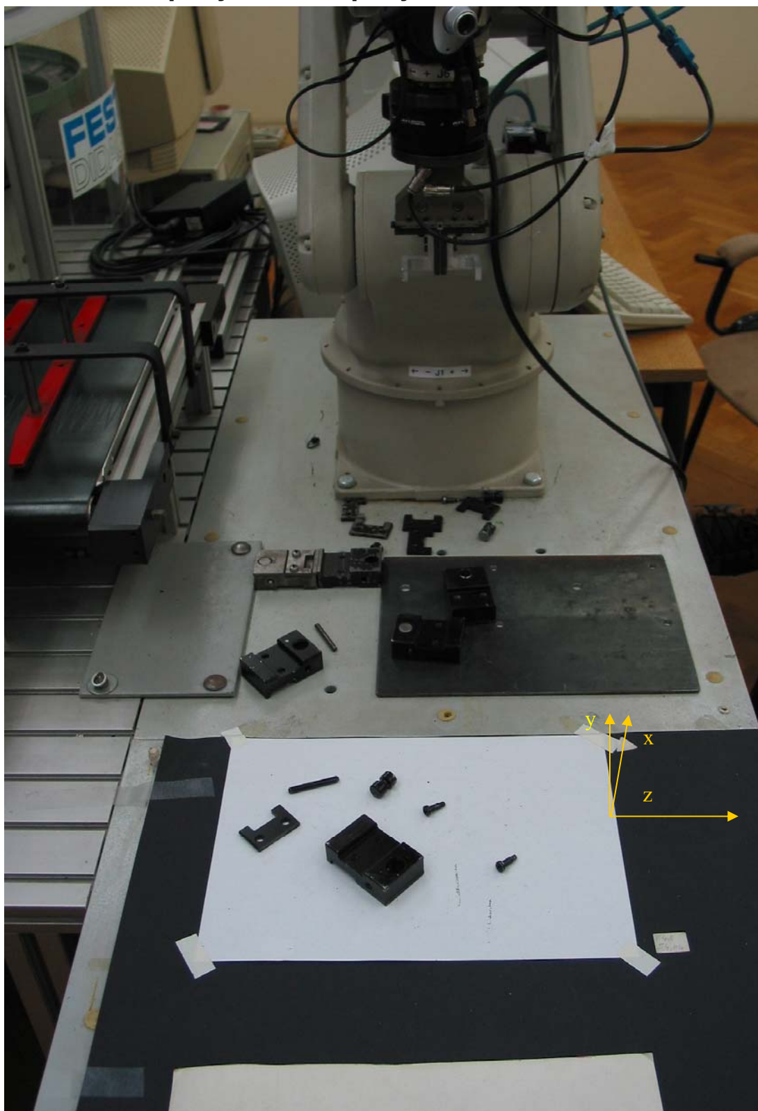
Slika 12. Robot i njegov radni prostor
